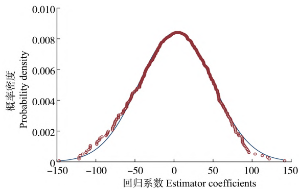
图 2 回归系数估计值的概率密度分布
